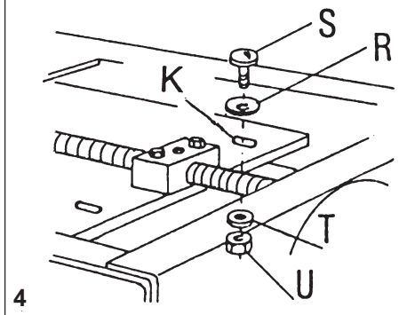
Valve upside down / Ansicht Schieber-Unterseite Vanne renversée / Valvola rovesciata
